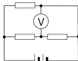
電路 (b)
