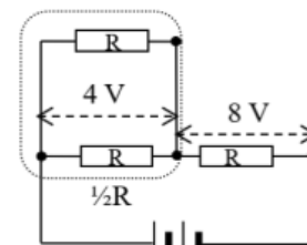
電路 (a)
